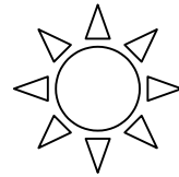
die Sonne
